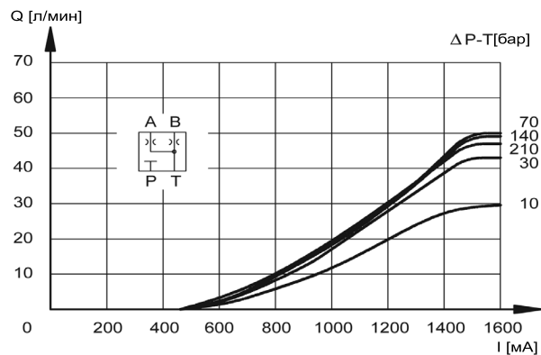
ТИП ЗОЛОТНИКА А30
