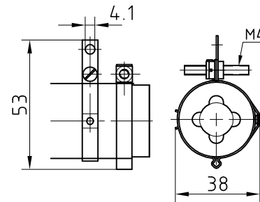
FZ / FU 100 x 35 F - FZ / FU 330 x 35 F mit Schraubschellen / with screw clips mit 1 Abgreifschelle / with 1 adjustable clip FZ / FU 100 x 35 F2 - FZ / FU 330 x 35 F2 mit 2 Abgreifschellen / with 2 adjustable clips FZ / FU 100 x 35 Fn - FZ / FU 330 x 35 Fn mit n Abgreifschellen / with n adjustable clips
