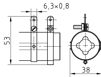
FZ / FU 100 x 35 ST - FZ / FU 330 x 35 ST mit Steckschellen / with fast - on clips mit 1 Abgreifschelle / with 1 adjustable clip FZ / FU 100 x 35 S2T - FZ / FU 330 x 35 S2T mit 2 Abgreifschellen / with 2 adjustable clips FZ / FU 100 x 35 SnT - FZ / FU 330 x 35 SnT mit n Abgreifschellen / with n adjustable clips
