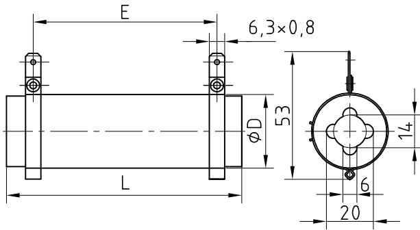
FZ / FU 100 x 35 S - FZ / FU 330 x 35 S mit Steckschellen / with fast - on clips ohne Abgreifschelle / without adjustable clip
