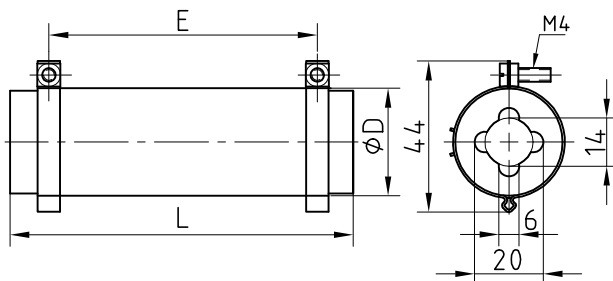
FZ / FU 100 x 35 - FZ / FU 330 x 35 mit Schraubschellen / with screw clips ohne Abgreifschelle / without adjustable clip
